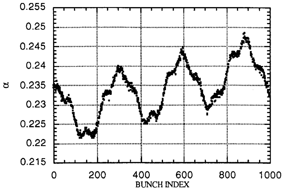
Figure 15: Twiss parameter \alpha [rad]
